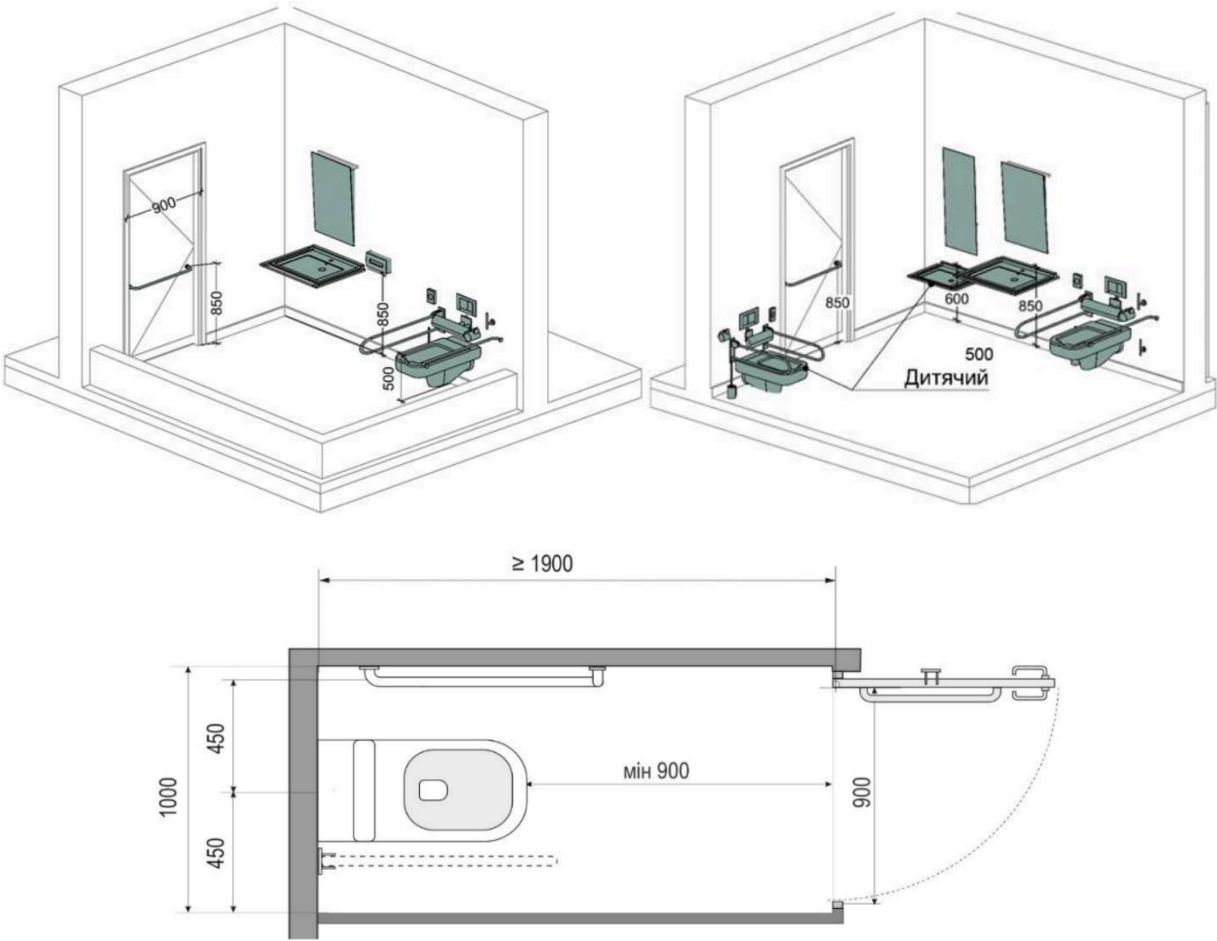
Малюнок 22 – Схематичне зображення варіантів окремого санітарно-гігієнічного приміщення для МГН
