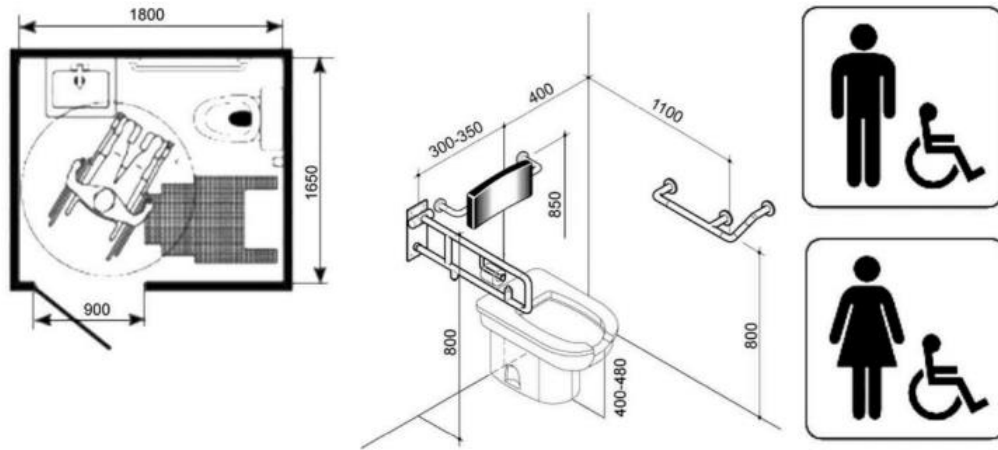
Малюнок 23 – Приклад обладнання універсальної kabіни (план, фрагмент облаштування унітаза поручнями)
