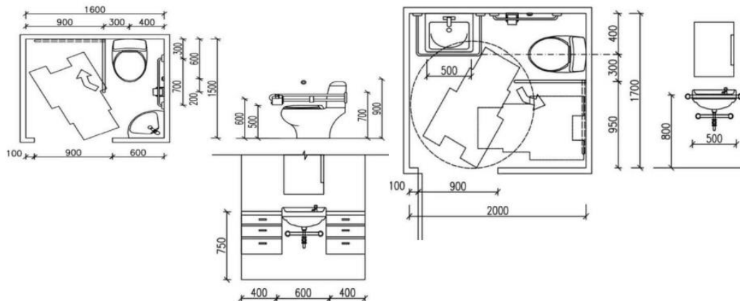
Малюнок 23 – Приклад обладнання універсальної kabіни (план, фрагмент облаштування унітаза поручнями)
