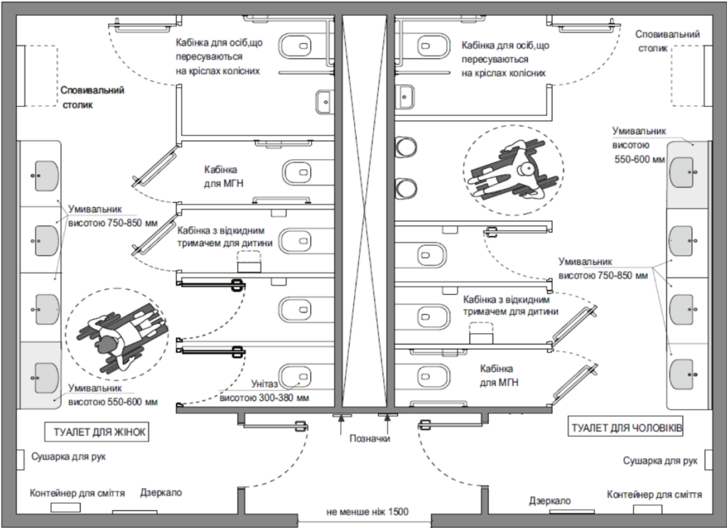
Малюнок 21 – Приклад облаштування універсальної кабіни в туалеті загального користування
