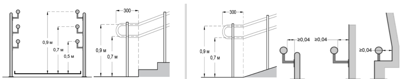
Малюнок 3 – Приклад влаштування поручнів в т.ч їх завершальної частини з прикладами кріплення
