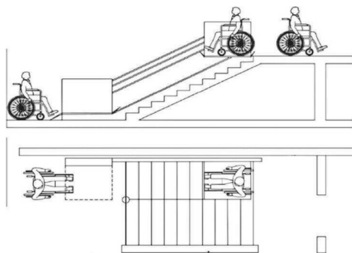
Малюнок 9 – Індивідуальні підйомники (похилі)
