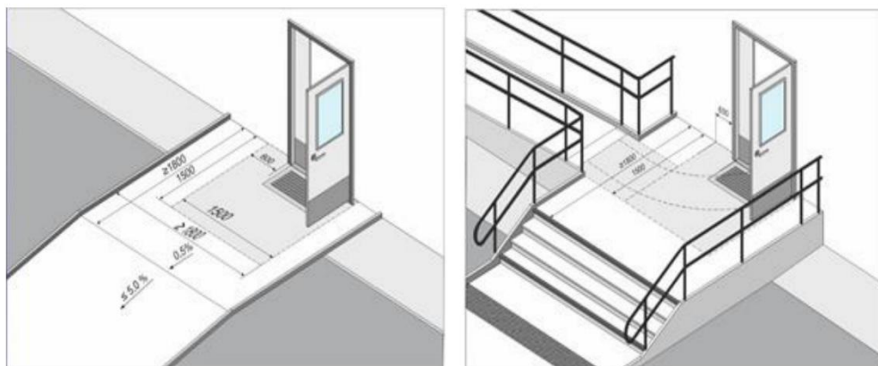
Малюнок 8 – Приклад влаштування вільного простору для маневрування перед вхідними дверима
