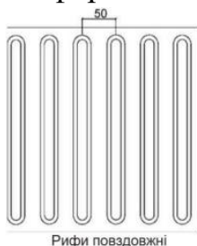
Малюнок 17 – Спеціальні тактильні індикатори (плити)
