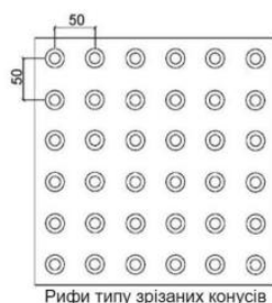
Малюнок 17 – Спеціальні тактильні індикатори (плити)
