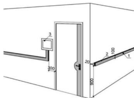
Малюнок 16 – Приклад улаштування ТІП приміщень за неможливості розміщення тактильної таблички справа від дверей
