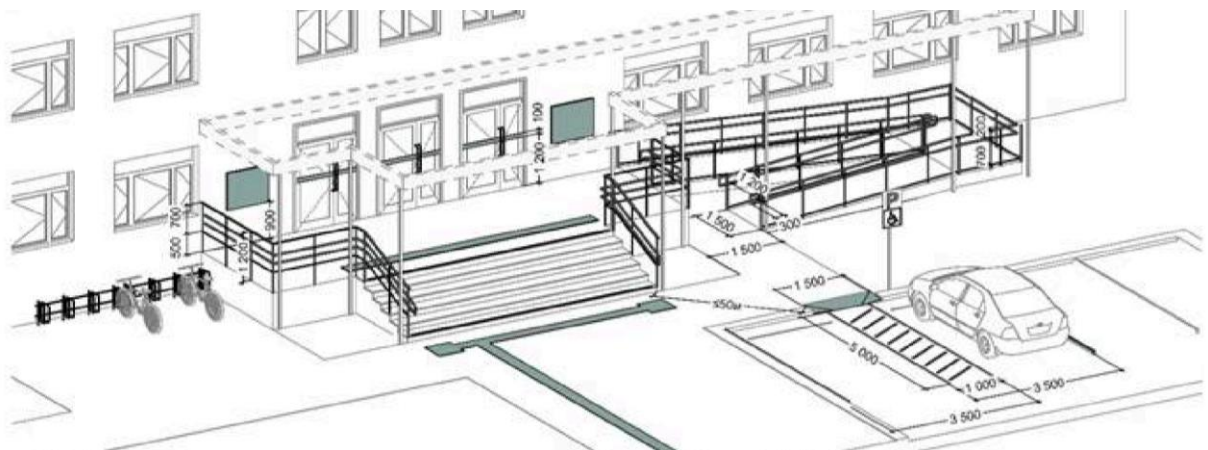
Малюнок 7 – Схематичне зображення вхідної групи до закладу освіти
