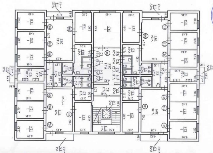
Фото 54 - Викопіювання з плану БТІ
