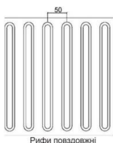
Малюнок 25 – Спеціальні тактильні індикатори (плити)
