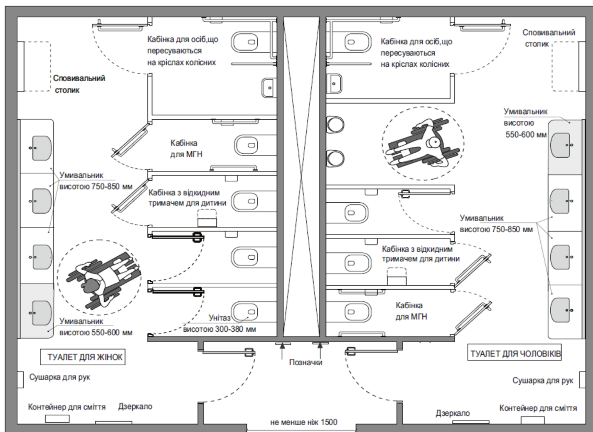
Малюнок 29 – Приклад облаштування універсальної кабіни в туалеті загального користування
