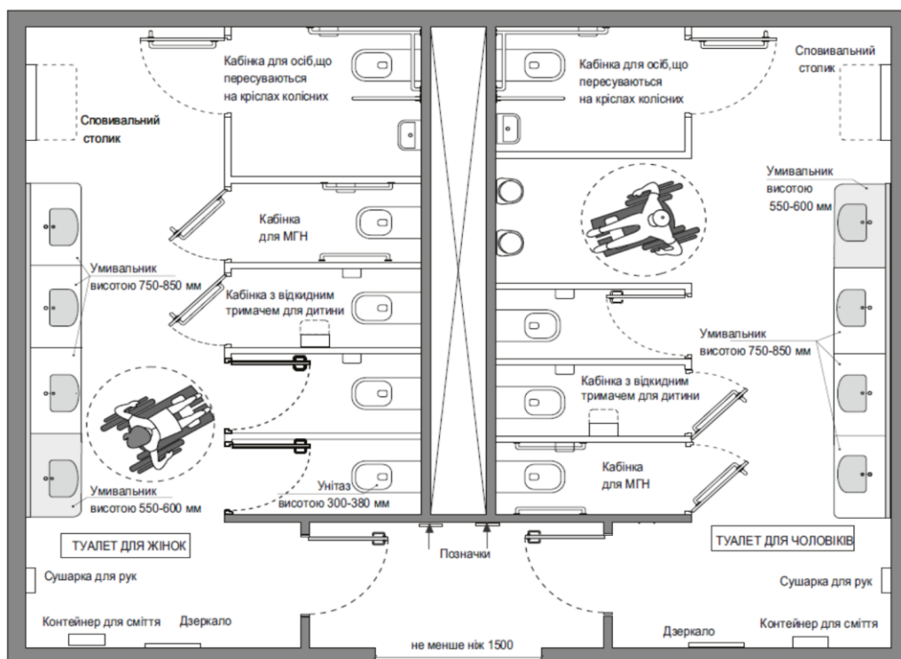
Малюнок 29 – Приклад облаштування універсальної кабінки в туалеті загального користування
