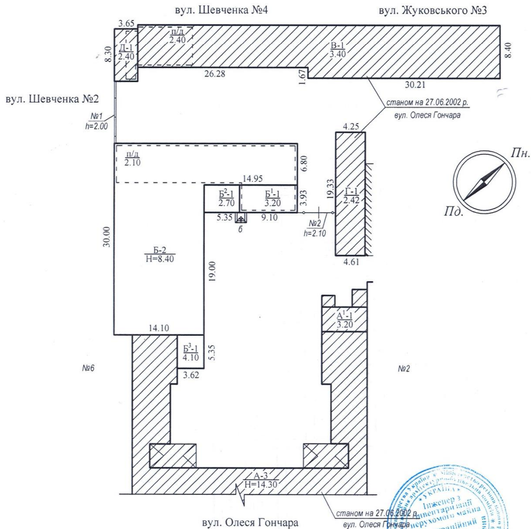
Малюнок 2 – Загальна схема території місця розміщення об'єкту
