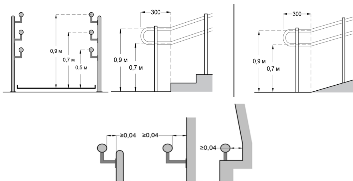
Малюнок 4 – Приклад влаштування поручнів в т.ч їх завершальної частини з прикладами кріплення
