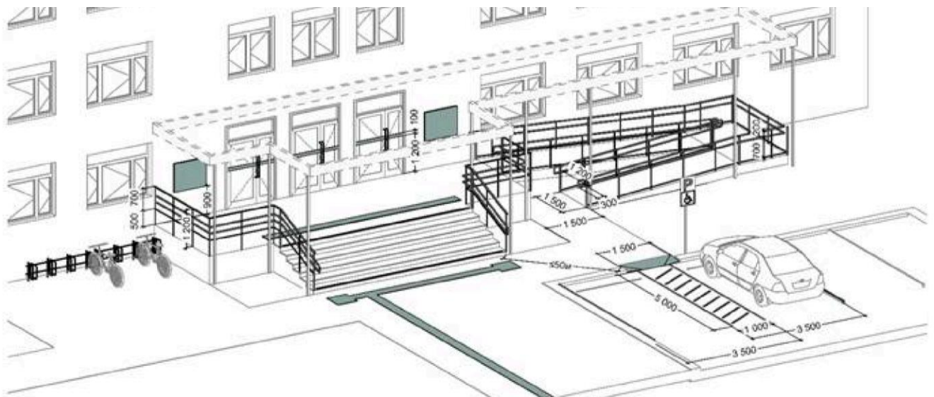
Малюнок 9 – Схематичне зображення вхідної групи до закладу освіти
