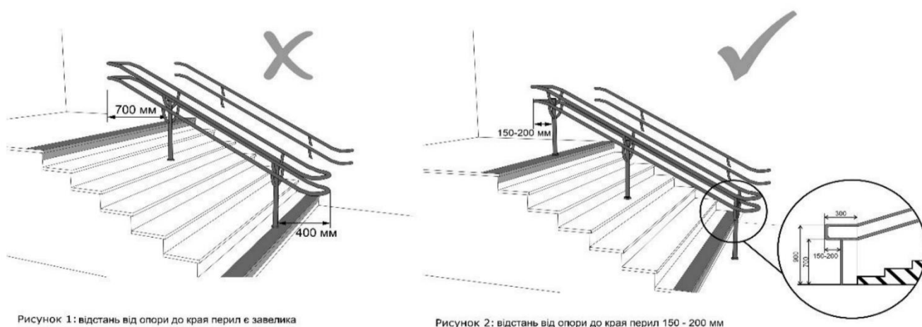
Малюнок 5 – Приклад влаштування першої та останньої опор поручнів
