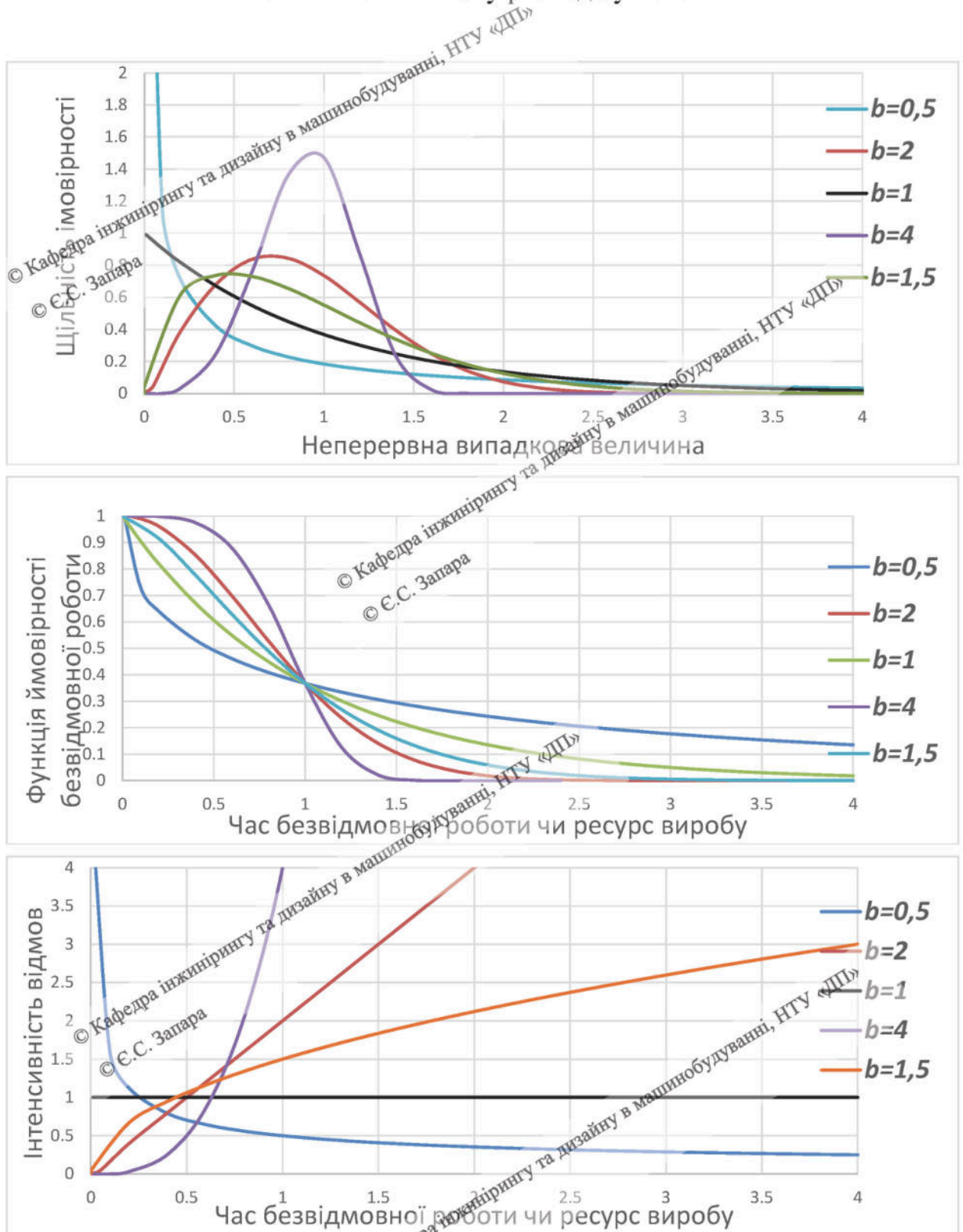
Рис. 3.19 Статистичні функції закону розподілу Вейбулла при параметрі масштабу a = 1 і різних значення параметра форми b
