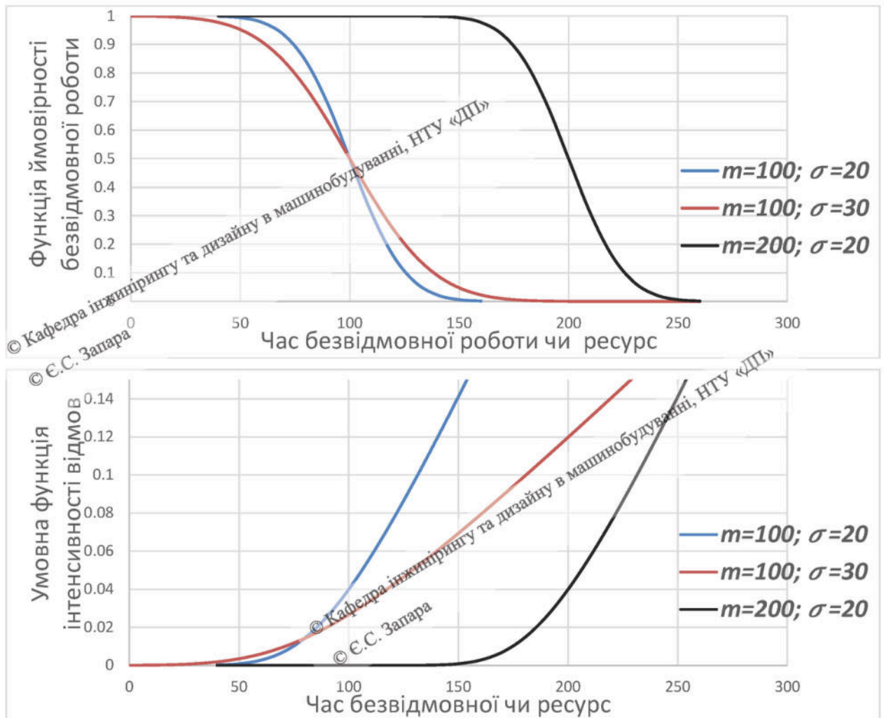
Рис. 3.14 Функції, що характеризують надійність машин при нормальному розподілі часу їх безвідмовної роботи
