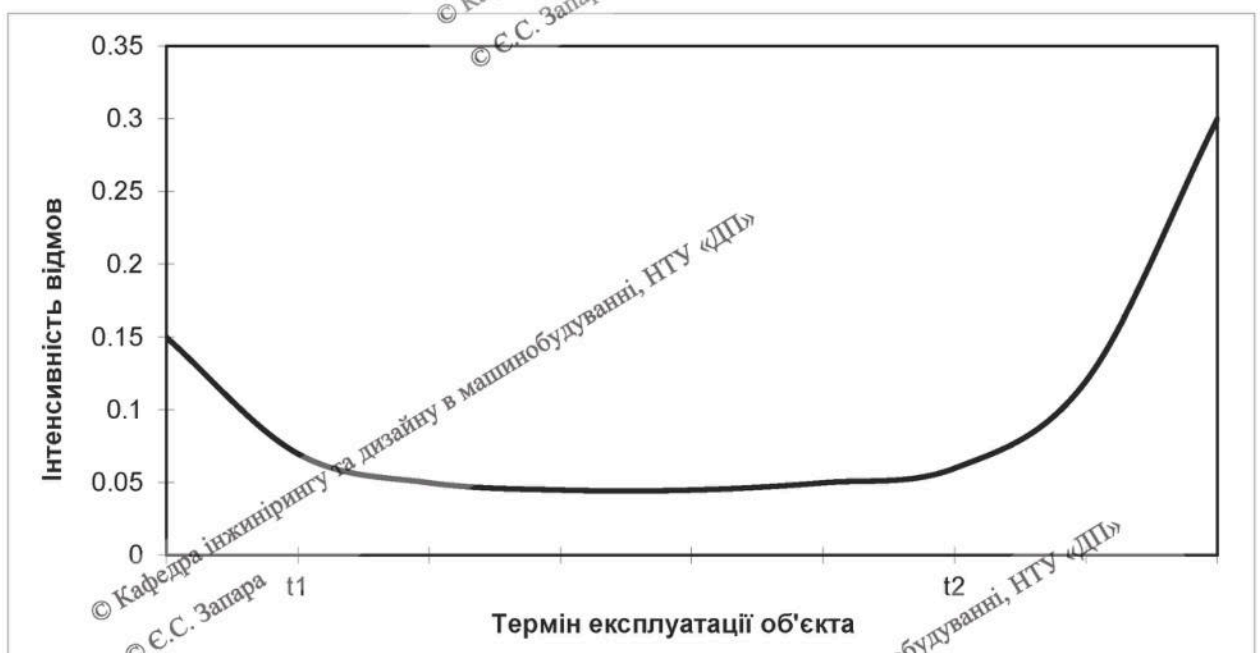
Рис. 3.10 Вид функції інтенсивності відмов, властивий більшості машин
