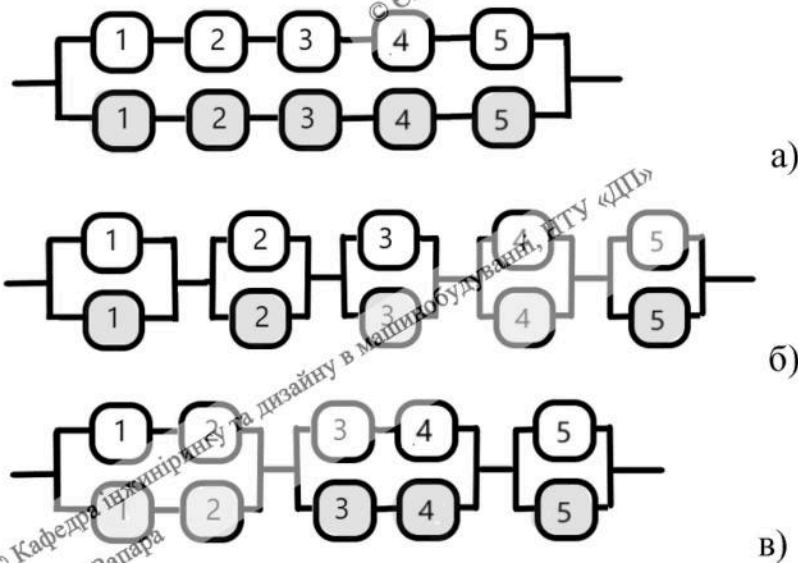
Рис. 5.4 Резервовані схеми з'єднання елементів у системі: а – загальне резервування; б – роздільне поелементне; в – роздільне групове
