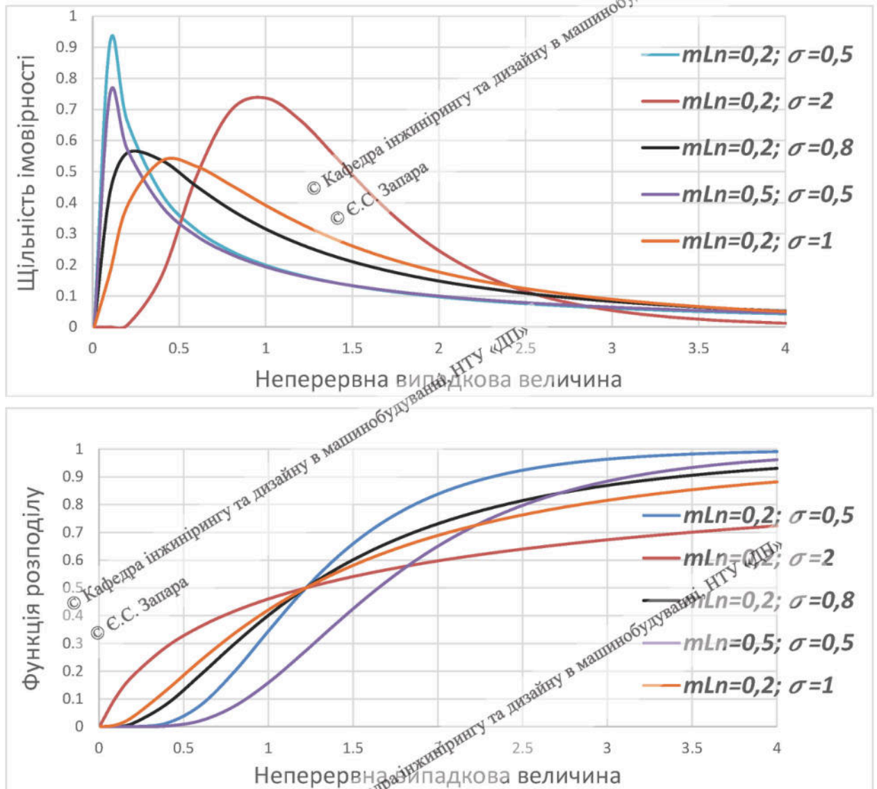
Рис. 3.15 Статистичні функції логарифмічно-нормального закону розподілу випадкових величин при різних параметрах
