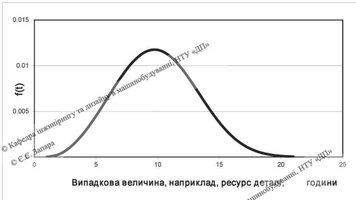
Рис. 3.4 Щільністю розподілу неперервної випадкової величини
