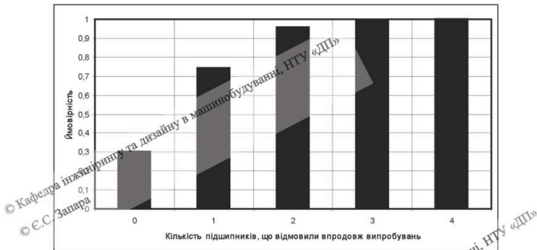
Рис. 3.2 Функція розподілу числа підшипників, що відмовили протягом ресурсних випробувань
