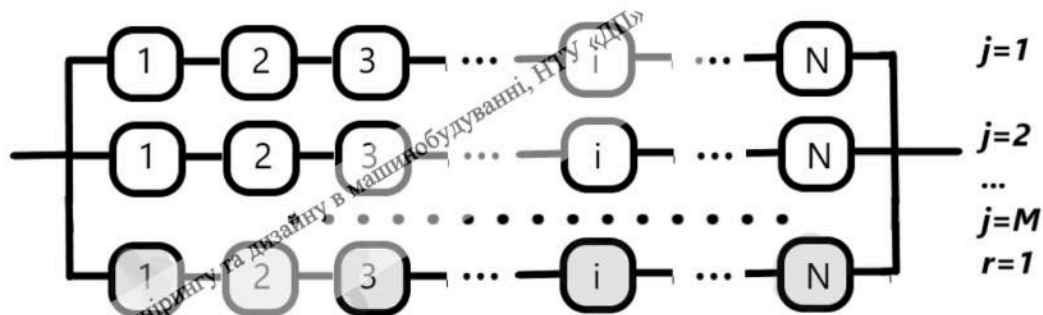
Рис. 5.3 Резервована схема з'єднання елементів системи. j – номер паралельної технологічної лінії, M – кількість основних ліній, r – кількість резервних ліній.
