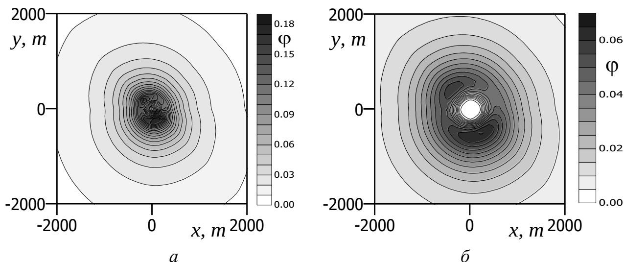
Рис. 3.6. Розподіл середньоїмовірної концентрації домішки \varphi (мг/м 3 ) на рівні землі при різній висоті джерела її викиду: a – 20 м, b – 50 м
