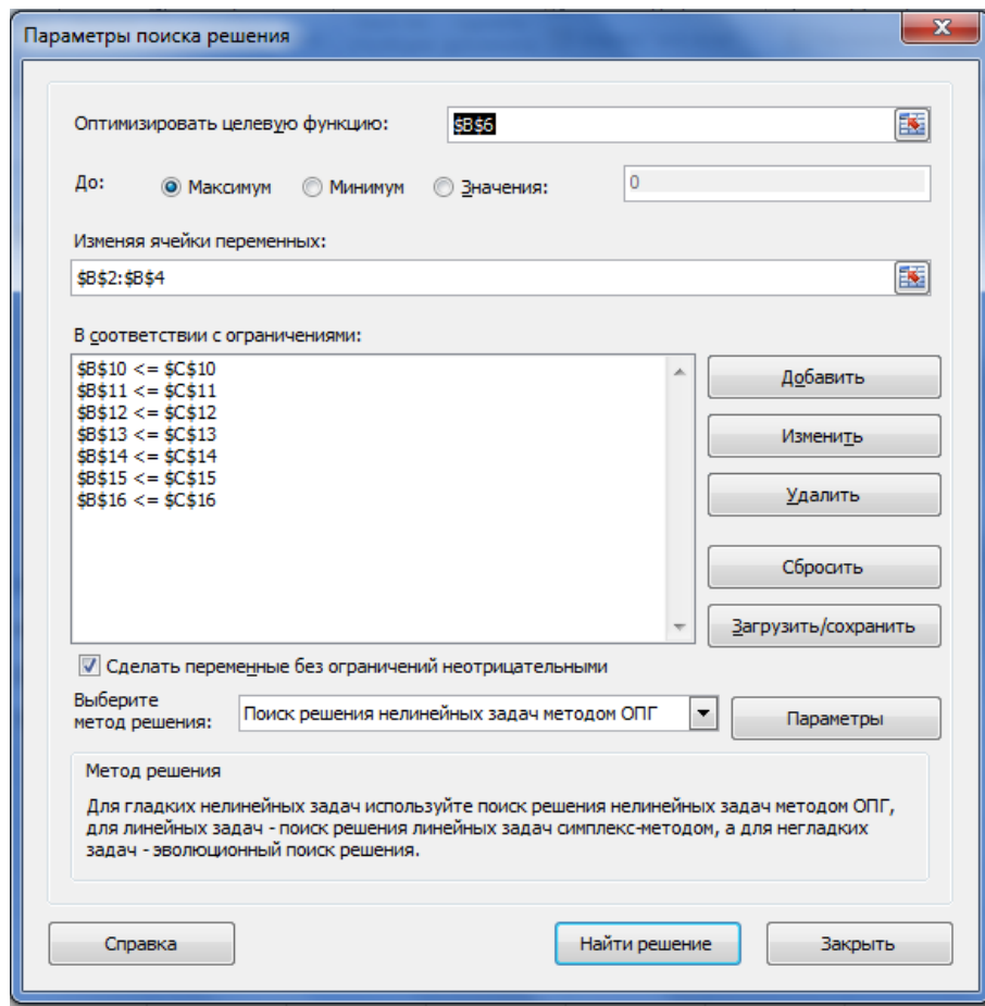
Рис. 5.6. Діалогове вікно для завдання параметрів оптимізації в програмі MS Excel
