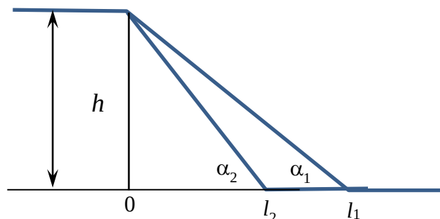
Рис. 4.2. Контур борту кар'єру при різних кутах нахилу
