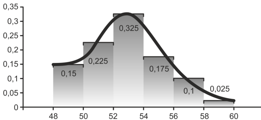
Рис. 2.8. Гістограма відносних частот межі міцності на стиск алевроліту (за даними табл. 2.6)
