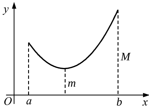
Рис. 4.4. Найбільше та найменше значення функції на відрізку
