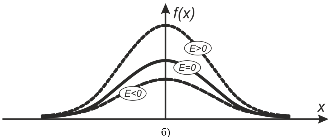
Рис. 2.9. Вигляд кривих щільності розподілу випадкової величини: а) при різній асиметрії, б) при різному ексцесі
