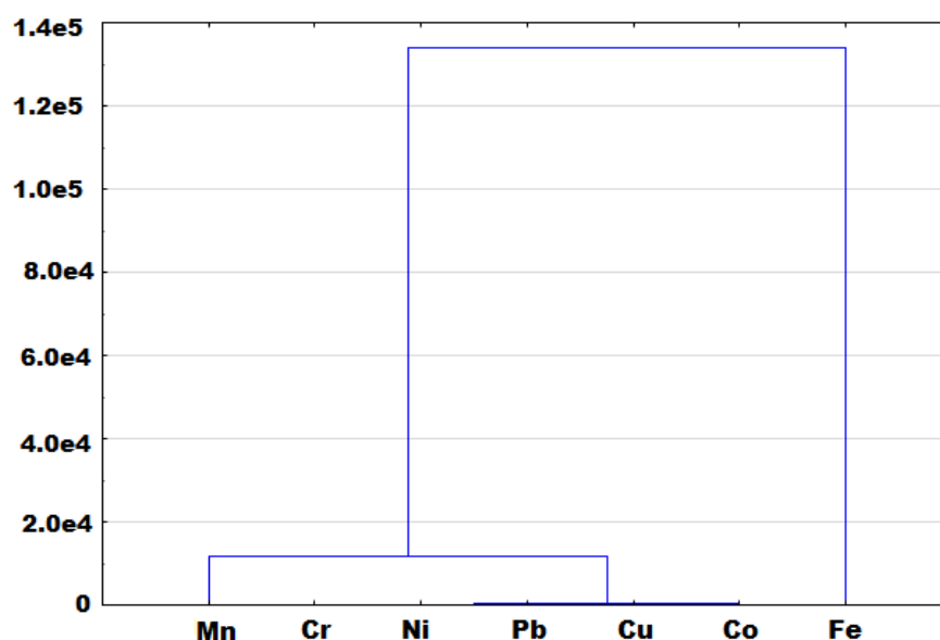
Рис. 3.20. Дендрограма геохімічних асоціацій важких металів (до прикладу 3.14)
