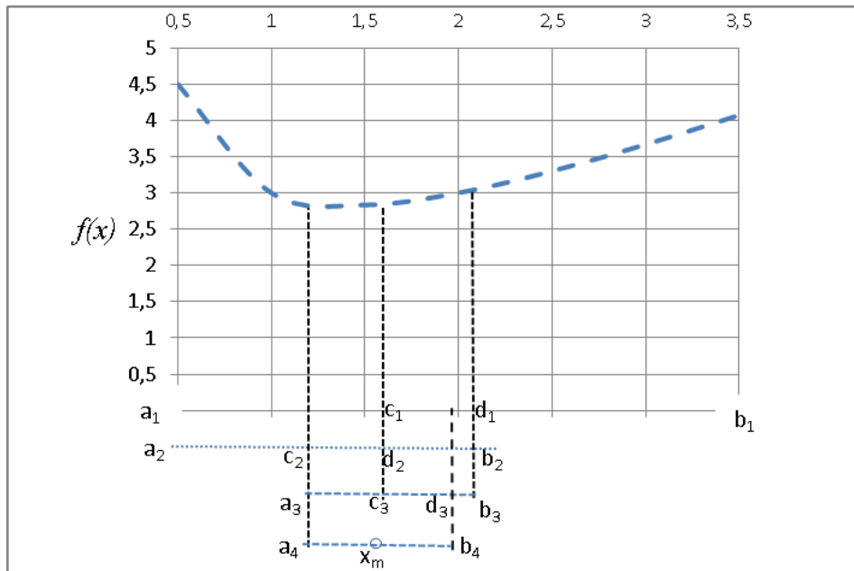
Рис. 4.9. Схема пошуку точки мінімуму за методом золотого перетину
