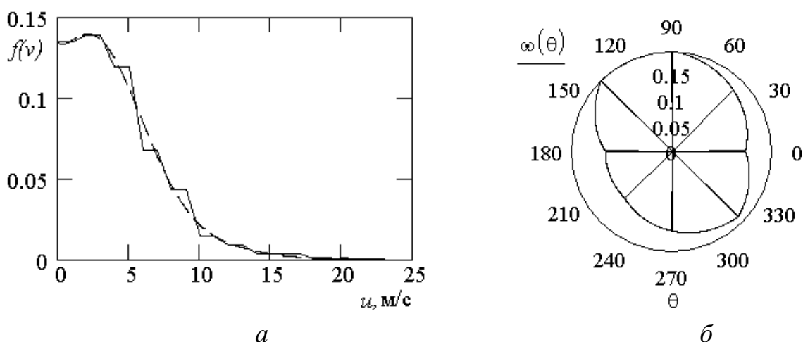
Рис. 3.5. Параметри вітрового режиму, використані в моделі: a – повторюваність швидкостей вітру ( — вимірювання, - - - апроксимація); b – роза вітрів
