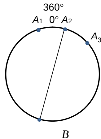
Рис. 3.3. Зображення вимірів азимутів кутів падіння прожилок у вигляді точок на окружності
