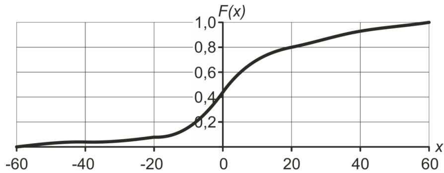
Рис. 2.3. Графік інтегральної функції для неперервної випадкової величини
