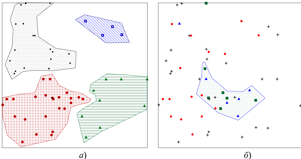
Рис. 3.16. Виділення кластерів на площині за критерієм геометричної близькості (а) та за вмістом рідкоземельного металу у пробі (б). Позначення: до 1 г/т (чорні маркери), 1 – 5 г/т (червоні маркери), 5 – 20 г/т (сині маркери), понад 20 г/т (зелені маркери)
