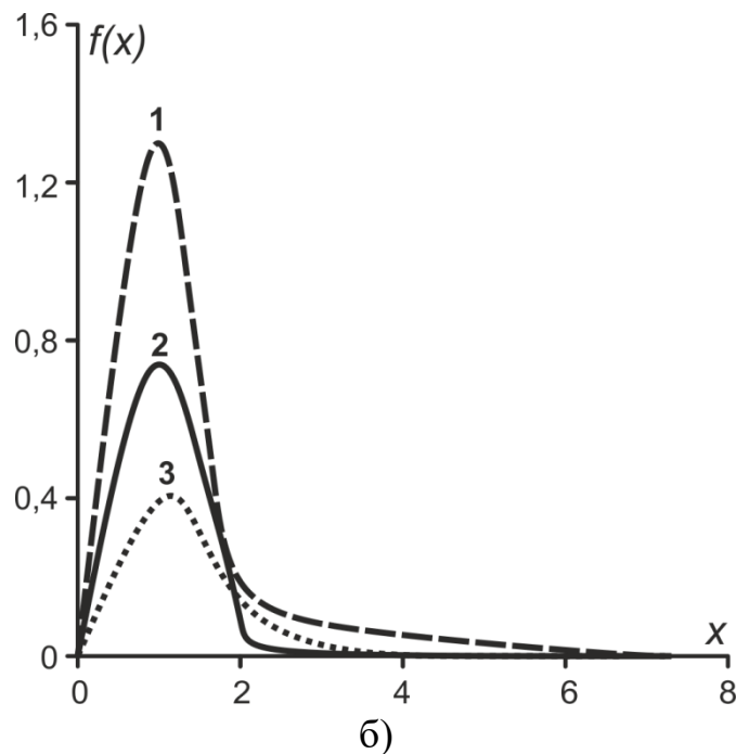
Рис. 2.15. Криві щільності логарифмічно нормального розподілу з різними значеннями параметрів: а) \sigma^2 = 1 при a = 0 (1), a = 0,3 (2) та a = 1 (3), б) a = 0 при \sigma^2 = 0,1 (1), \sigma^2 = 0,3 (2), \sigma^2 = 1 (3)
