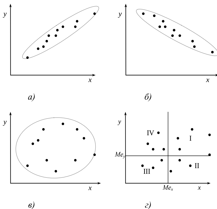
Рис. 2.23. Види кореляційного поля: а – прямий зв'язок між даними, б – зворотний зв'язок, в – зв'язок відсутній, г – схема до наближеного визначення коефіцієнта кореляції
