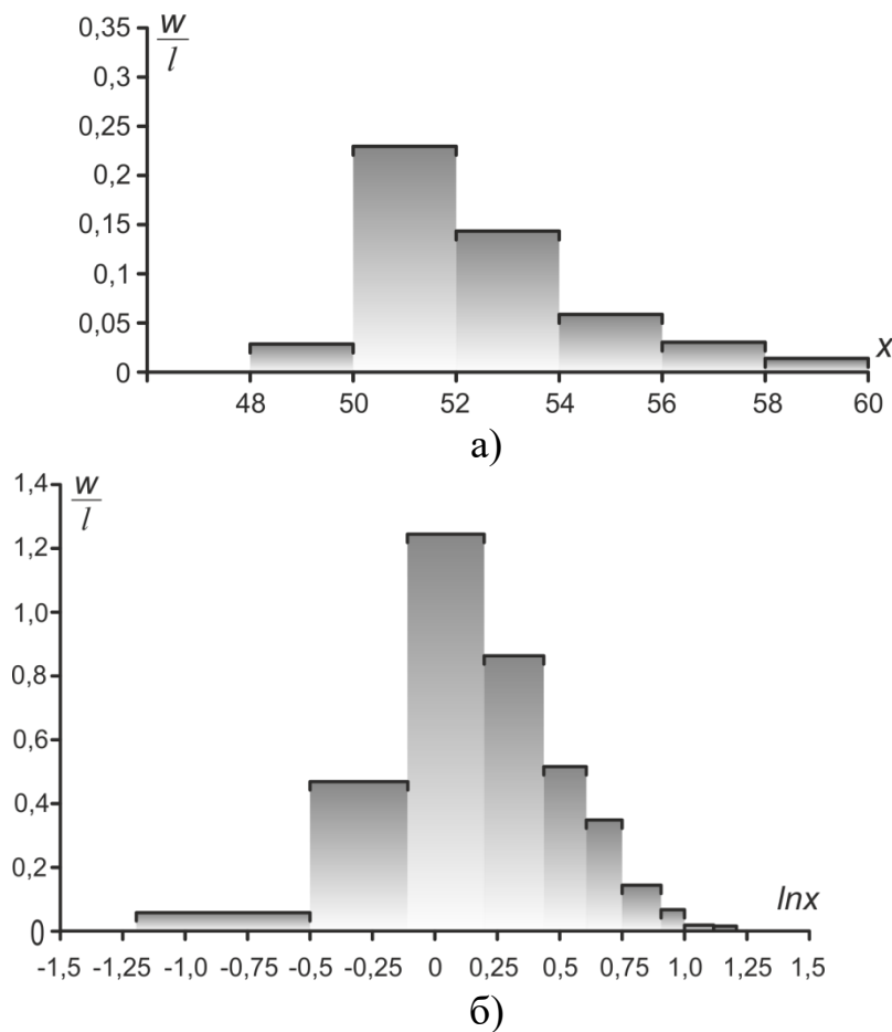
Рис. 2.14. Гістограма відносних частот потужностей пласта (а) та логарифмів потужностей пласта (б)
