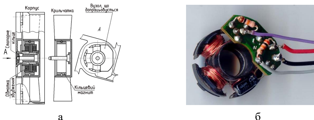
Рисунок 4.10 – Конструкція (а) та зовнішній вигляд модернізованої друкованої плати керування вентилятора HA4010V4 (б).
