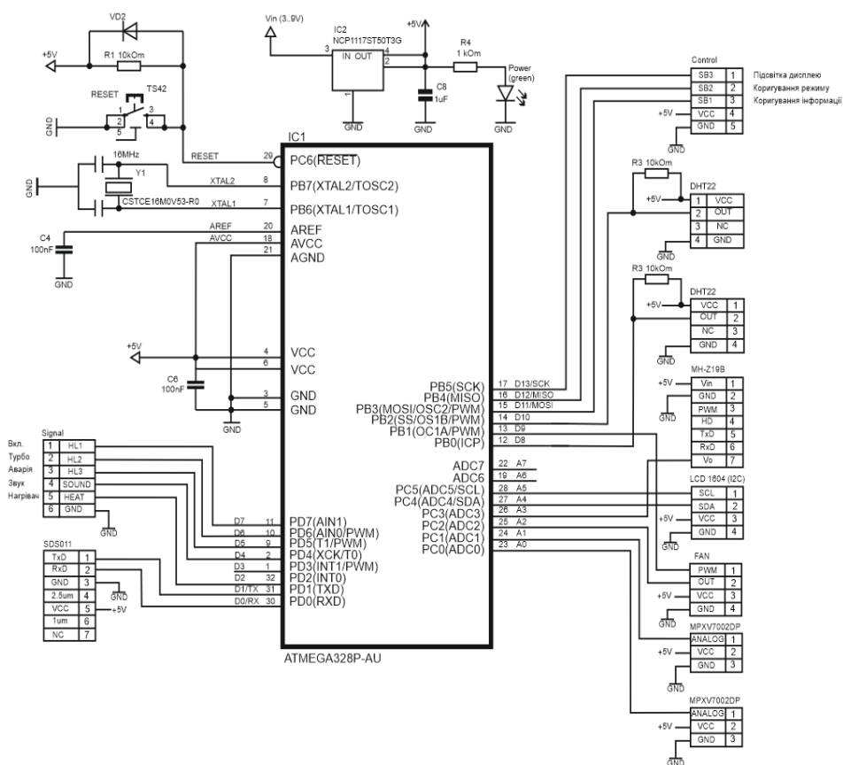
Рисунок 4.9 – Принципова електрична схема блоку контролера "Arduino Uno R3 Strong" [44]
