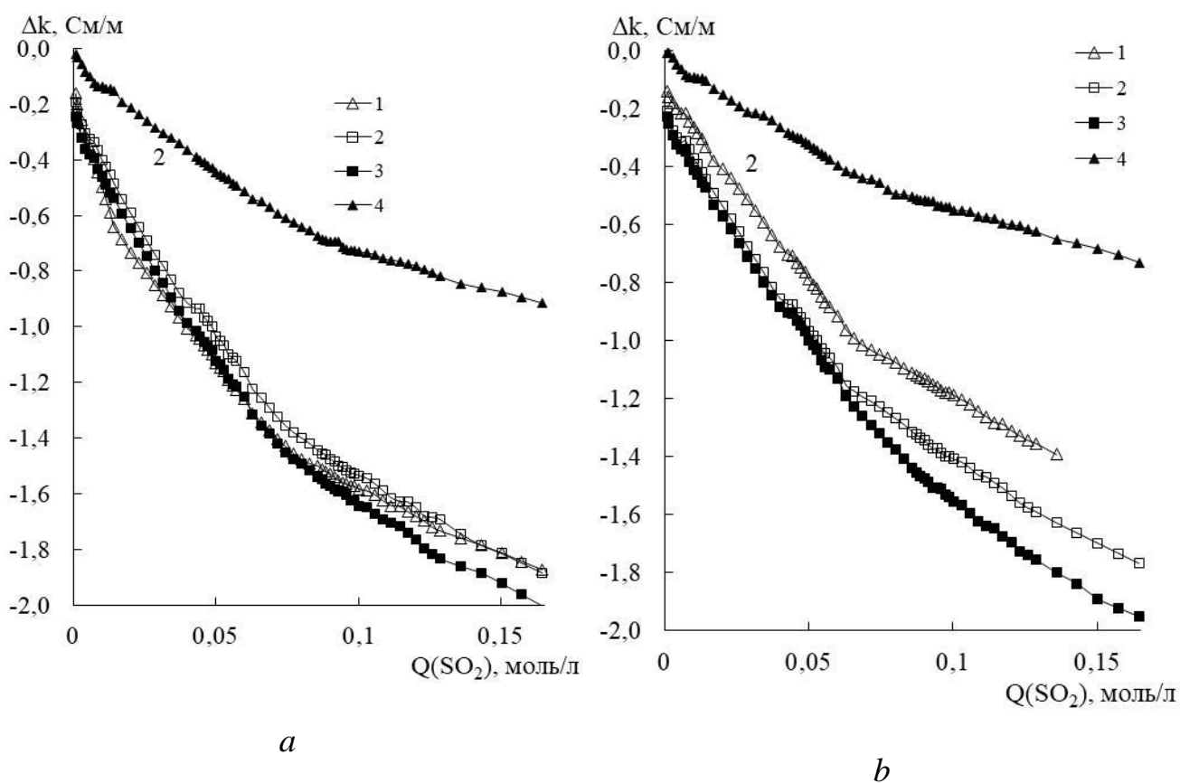
Рисунок 3.4 – Кондуктометричні криві титрування водних 0,1 М розчинів ТауК (а) та ТауМЕА (b) газоподібним \text{SO}_2 . Т (К): 298 – 1; 303 – 2; 308 – 3; 313 – 4.
